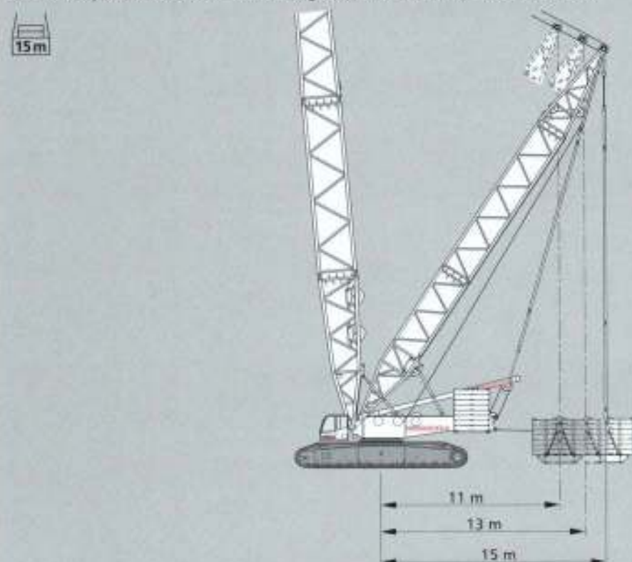
Standard Superlift attachment - serienmäßige Superlifteinrichtung - Superlift de série
