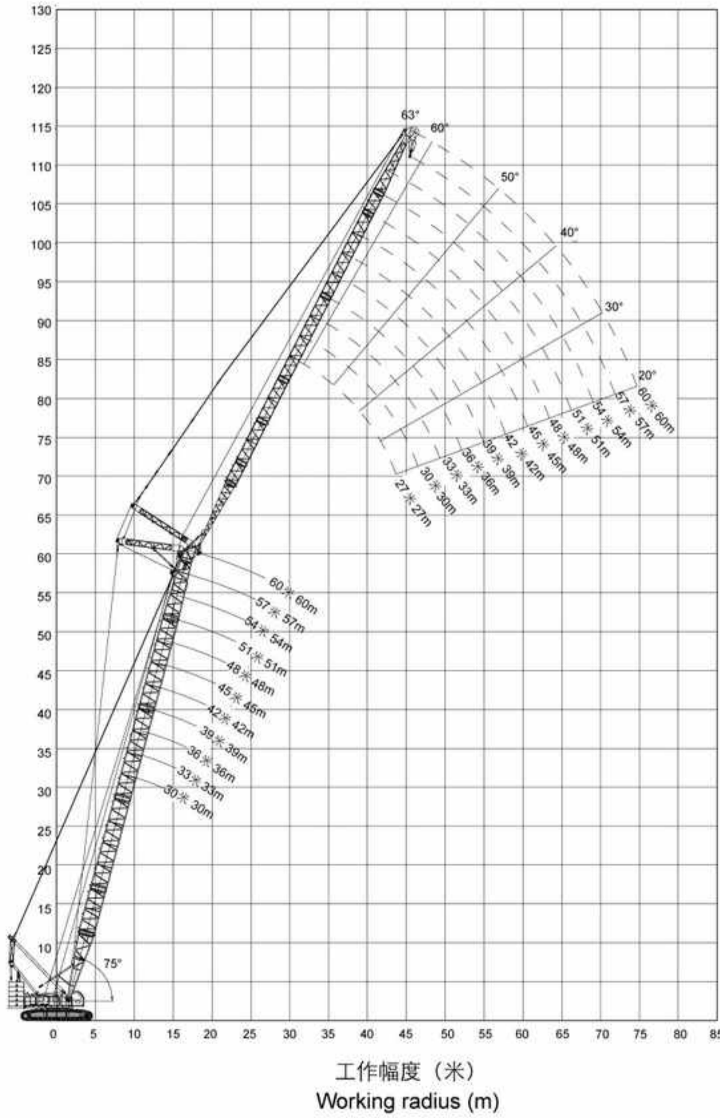
主臂75°时 Boom angle at 75°
