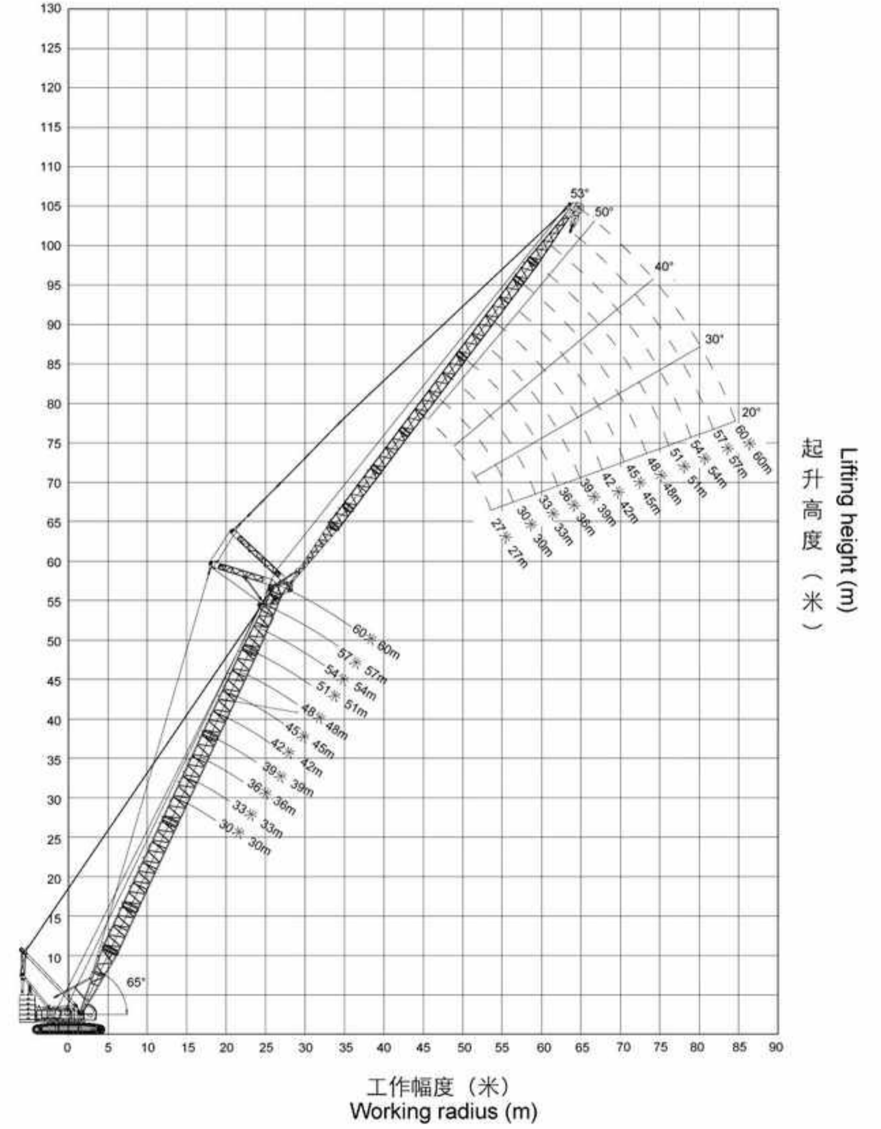
主臂65°时 Boom angle at 65°
